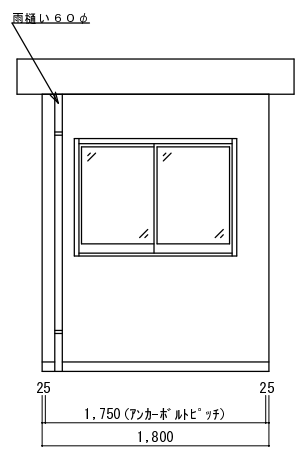
A 立面図
