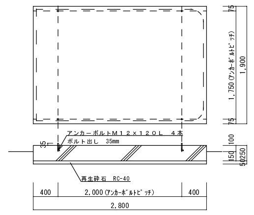
基礎図 (参考)
