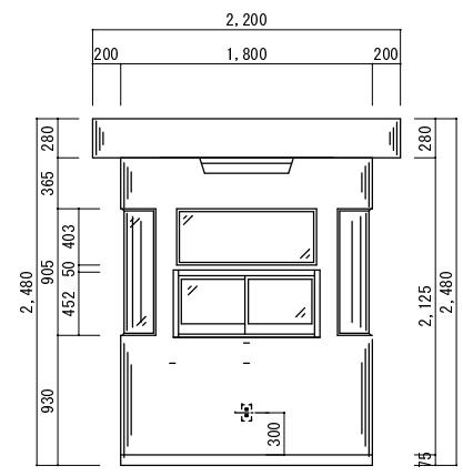
C 立面図
