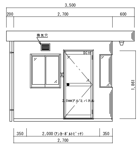
B 立面図
