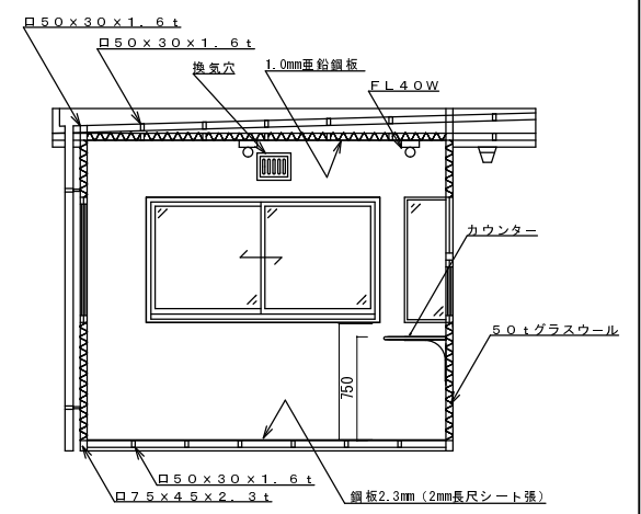
D 断面図
